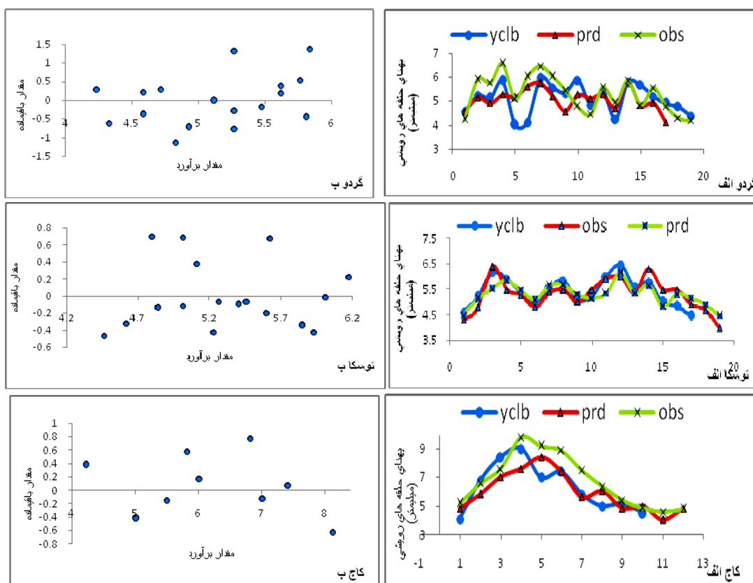
شکل ۶- مقادیر واقعی (obs)، برآورد (prd) و کالیبراسیون (yclb) در مدل‌های نهایی برای سه گونه گردو، توسکا ییلاقی و کاج بروسیا در طول سال‌های مورد نظر (الف) و مقدار باقی مانده کالیبراسیون در مقابل مشاهدات (ب)
