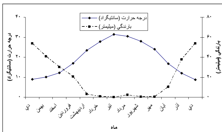
شکل ۱- نمودار بارش دمای (آمبروترمیک) جهرم
