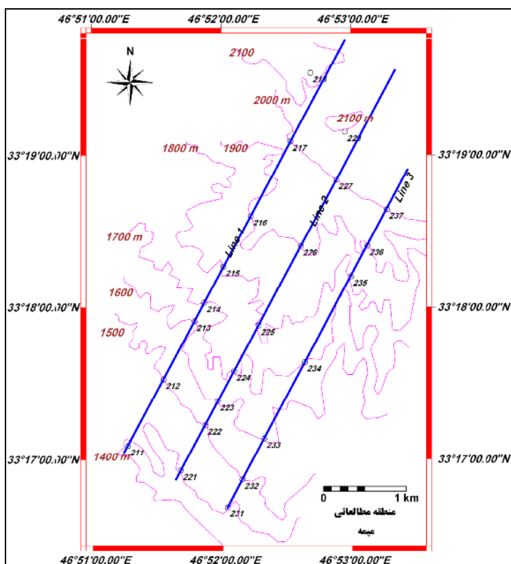
شکل ۲- موقعیت مناطق نمونه‌برداری در منطقه میمه
