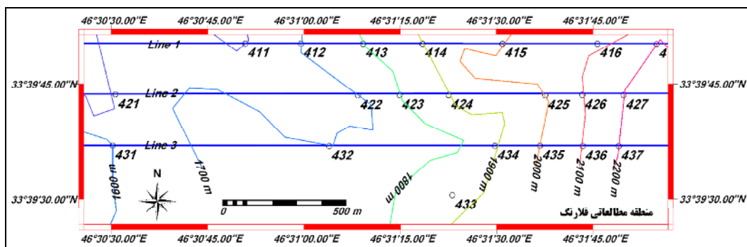
شکل ۱- نقشه موقعیت مناطق نمونه‌برداری در منطقه قلارنگ
