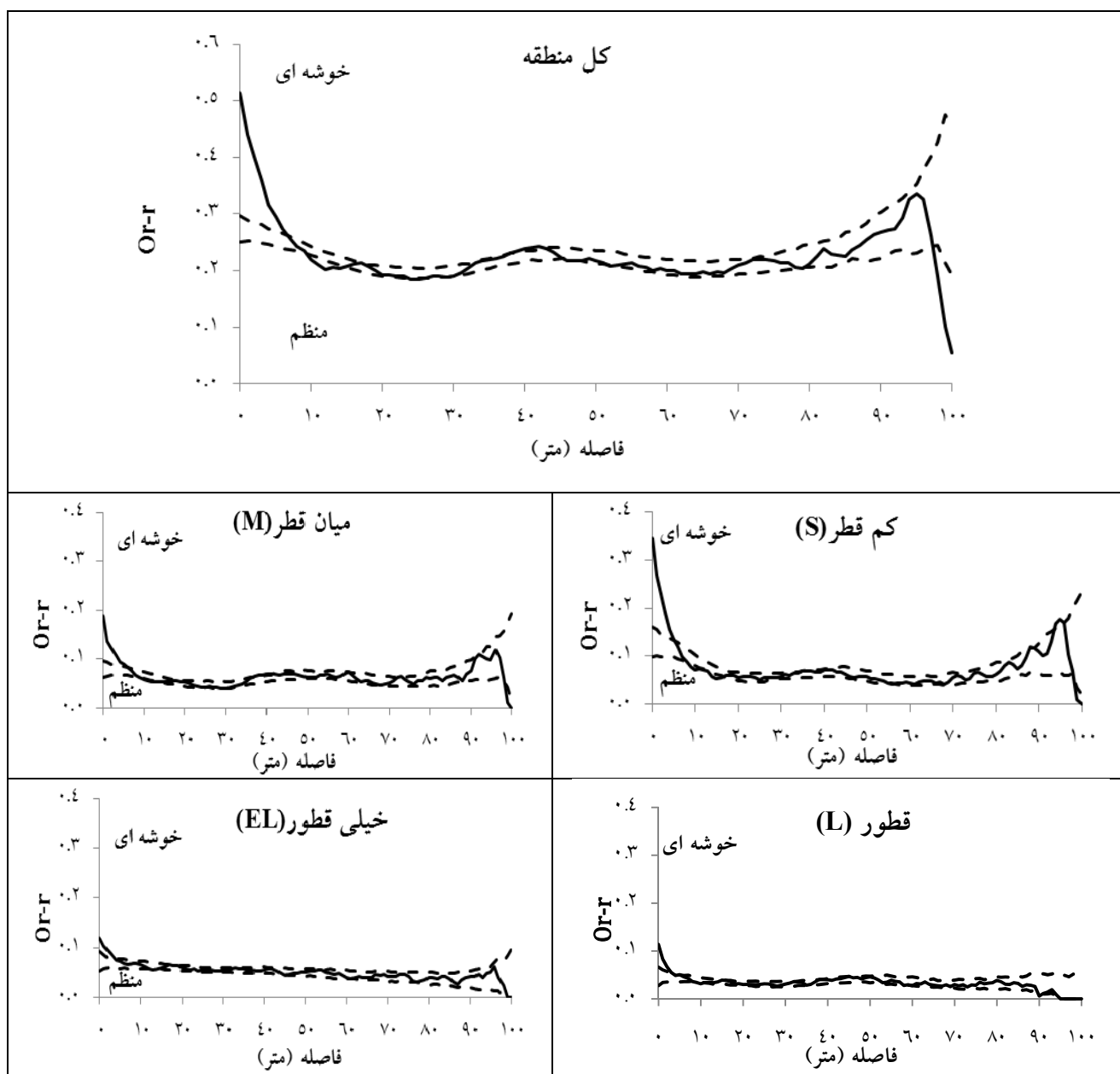
شکل ۲- نمودار آماره O_{12}(r) و حدود مونت کارلو (محدوده خط چین) در کل منطقه به تفکیک طبقه‌های قطری. حدود مونت کارلو محدوده فرض صفر یا الگوی پراکنش تصادفی را نشان می‌دهد.
