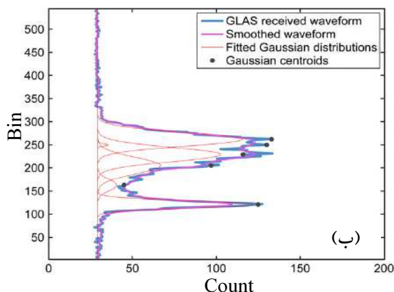
شکل ۳- نمونه ای از شکل موج ارسال شده (الف) و شکل موج دریافت شده (ب); در شکل ب شکل موج نرم شده و توزیع گوسی برازش شده نیز نشان داده شده است (Chen, 2010b).
