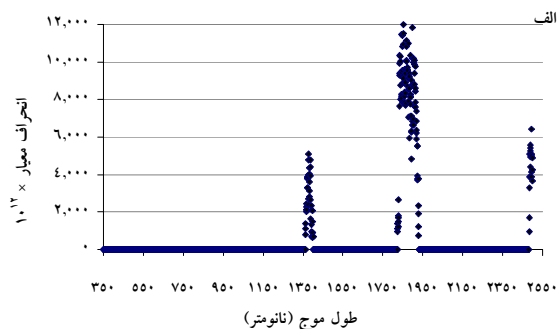
شکل ۶- انحراف معیار انعکاس طیفی محاسبه شده برای تمامی طول موج‌ها (الف)، منحنی بازتاب طیفی یک گونه پس از حذف بازتاب‌های دارای خطا (ب)
